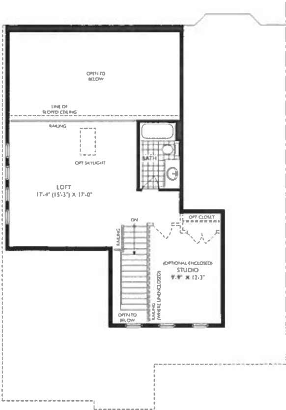
Optional Loft #1 597 sq.ft
